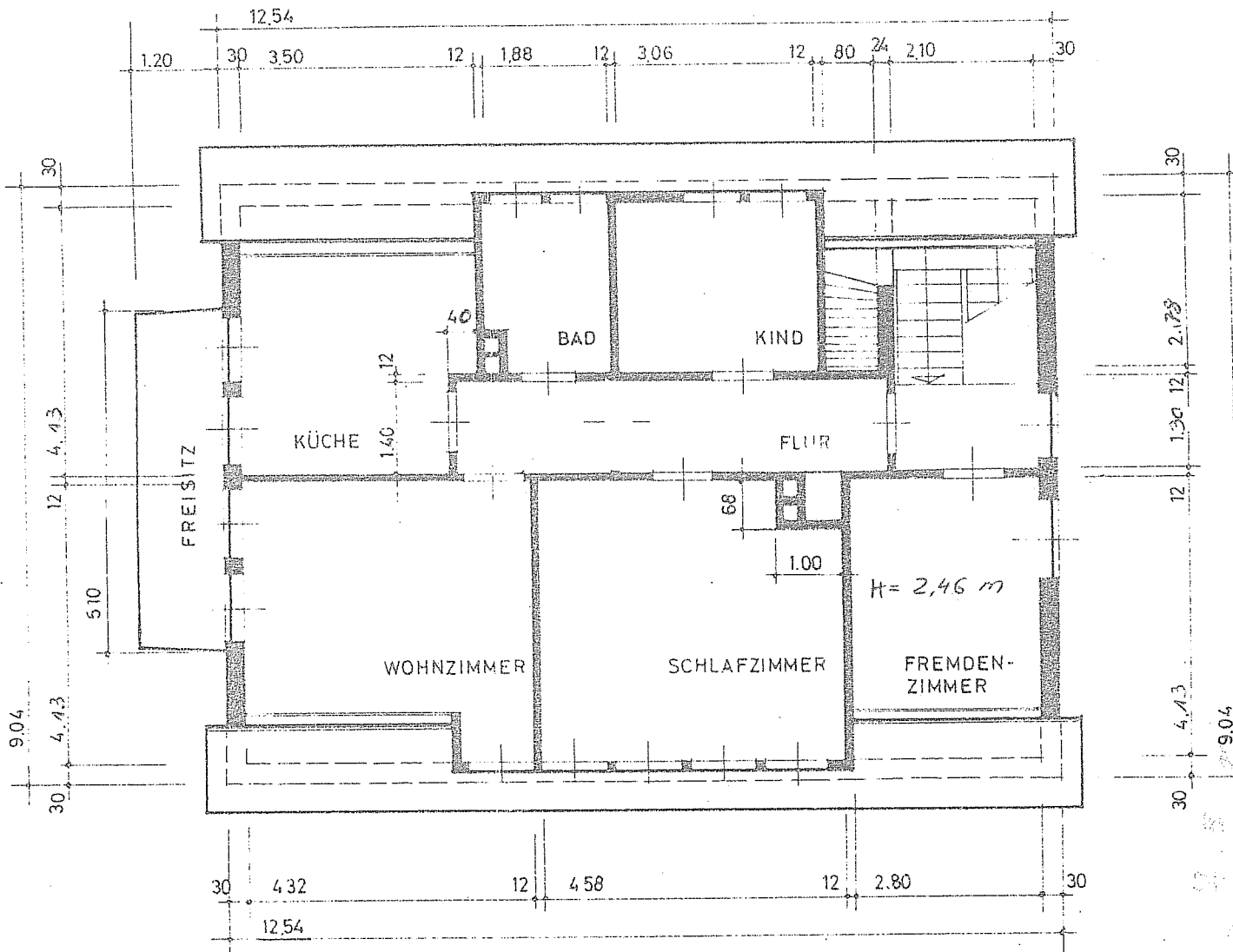
OBERGESCHOSS
