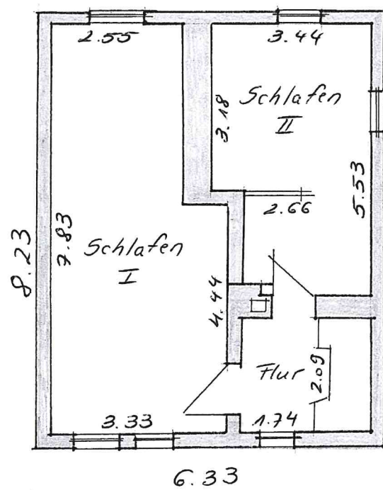
Obergeschoss
