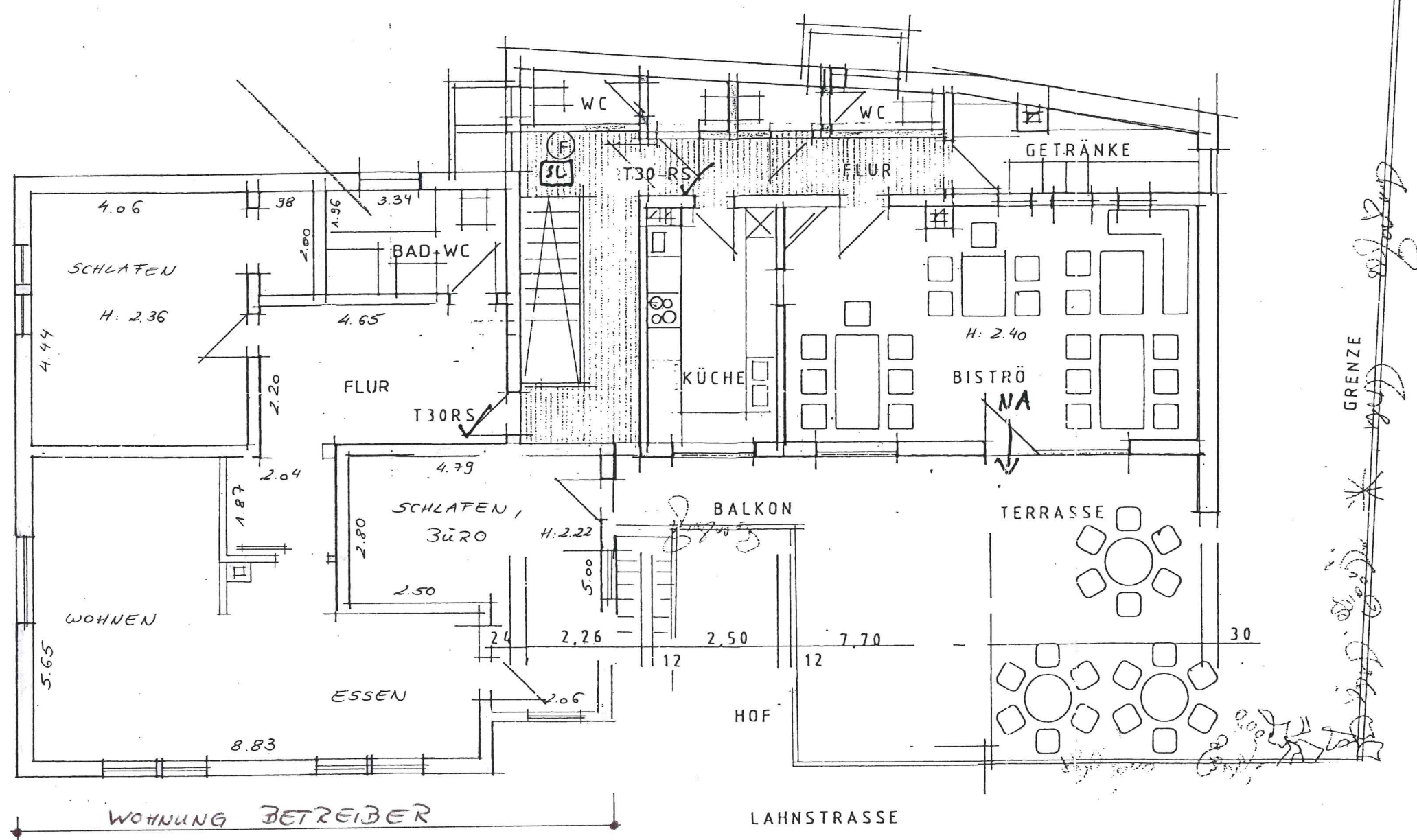
ERDGESCHOSSGRUNDRISS, M. 1:100
