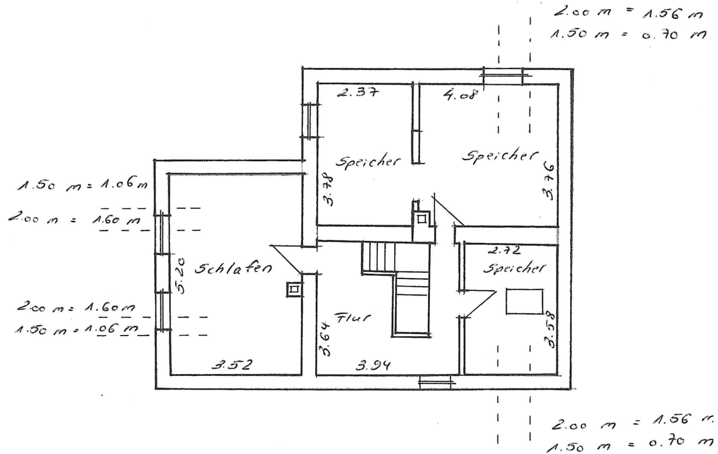
GRUNDRISS DACHGESCHOSS
