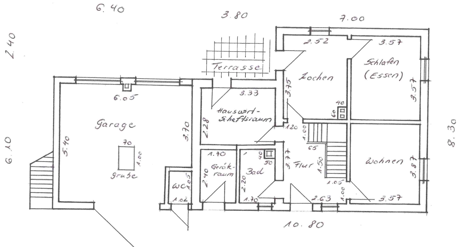
GRUNDRISS ERDGESCHOSS
