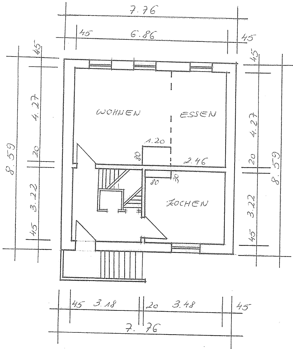
ERDGESCHOSS
