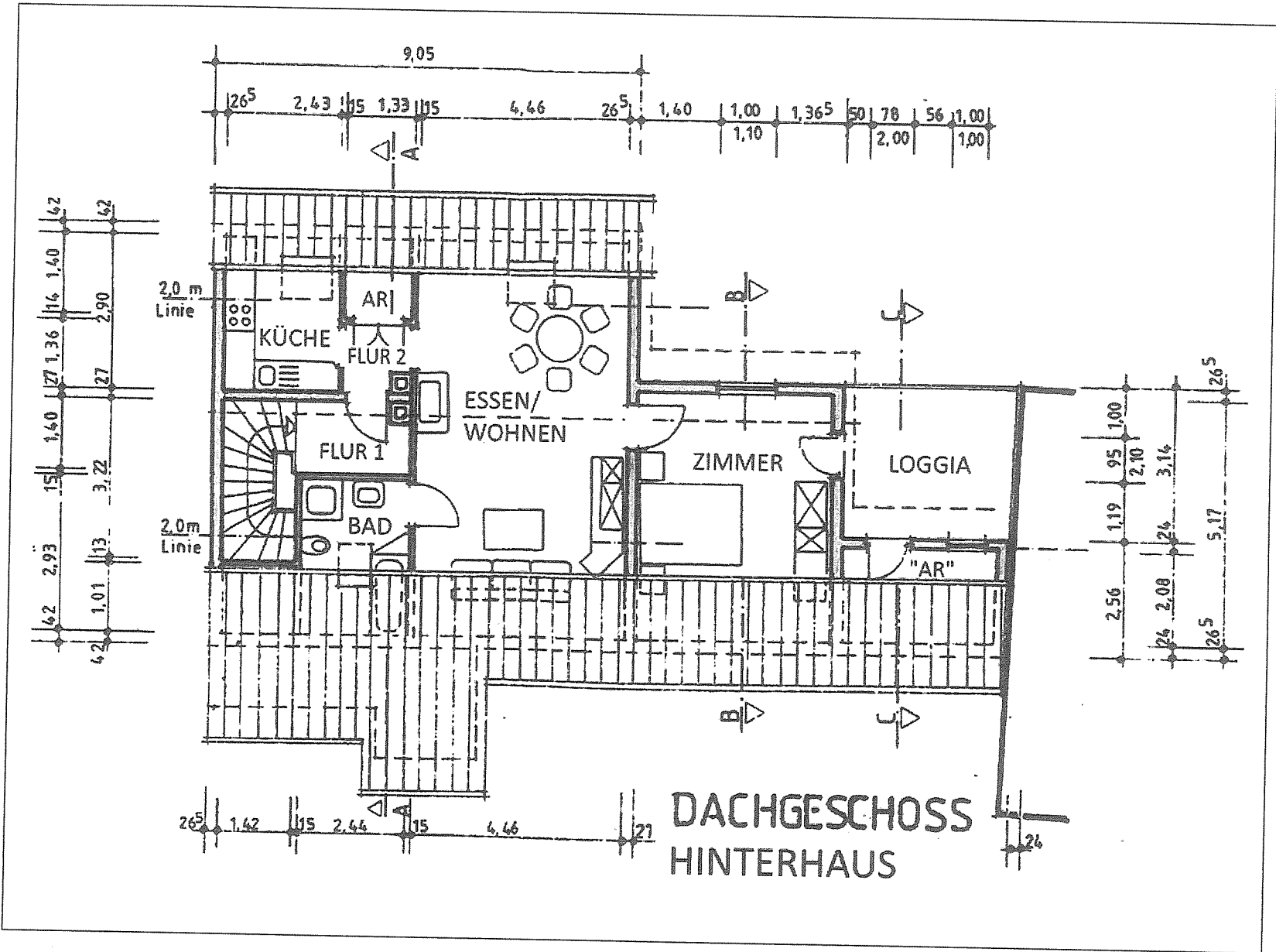
Dachgeschoss Hinterhaus
